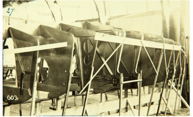
Fokker B.II en proceso de construcción (Foto archivo San Diego Air & Space Museum)
