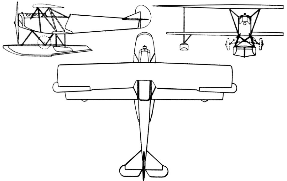
Fokker S.IIIW (Mercedes D-II de 120 hp)
