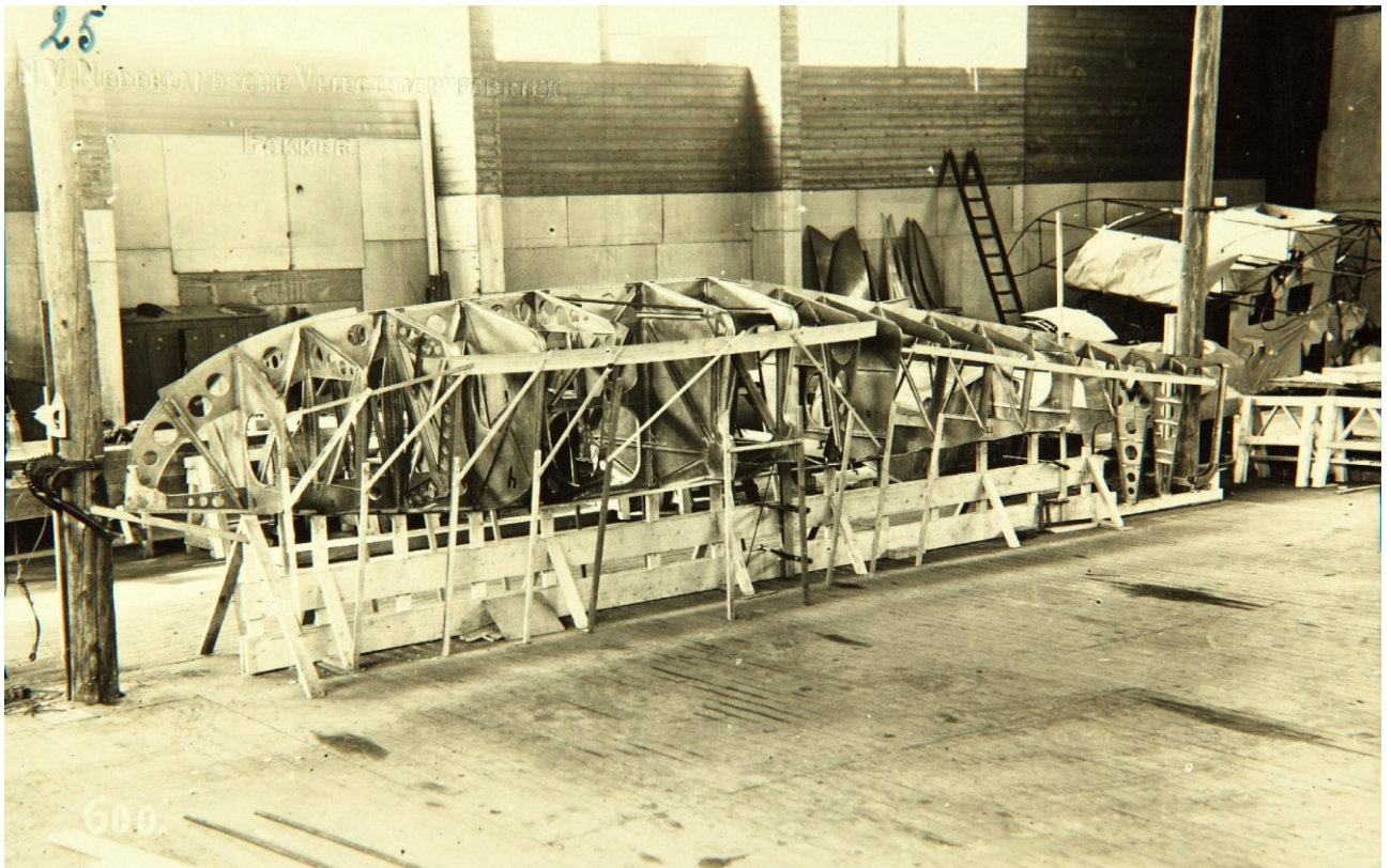
Fokker B.II en proceso de construcción (Foto archivo San Diego Air & Space Museum)
