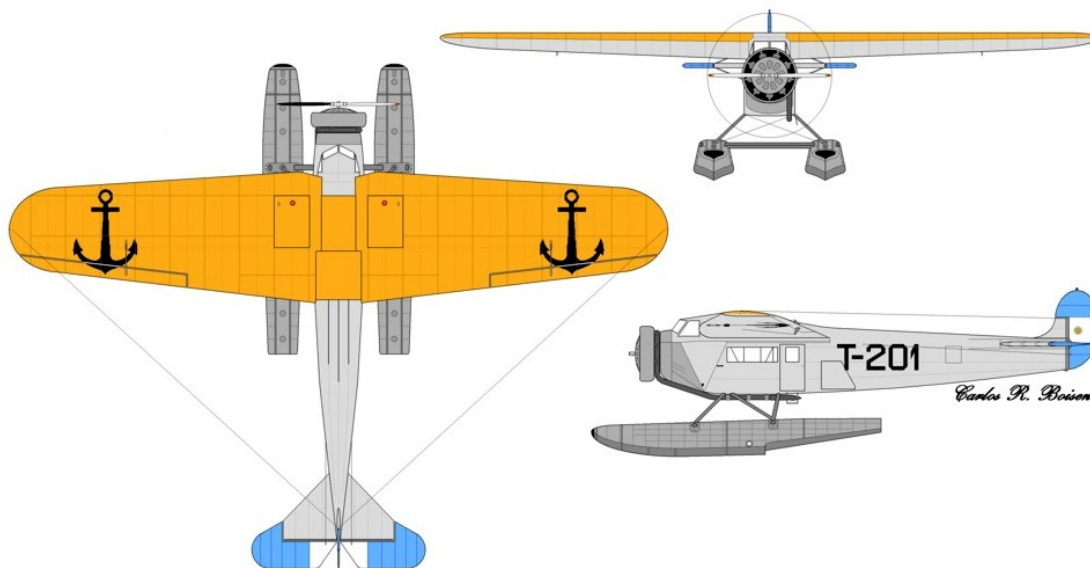
Fokker T-201 (ilustración de Carlos R. Boisen. Archivo Museo de Aviación Naval) 57
