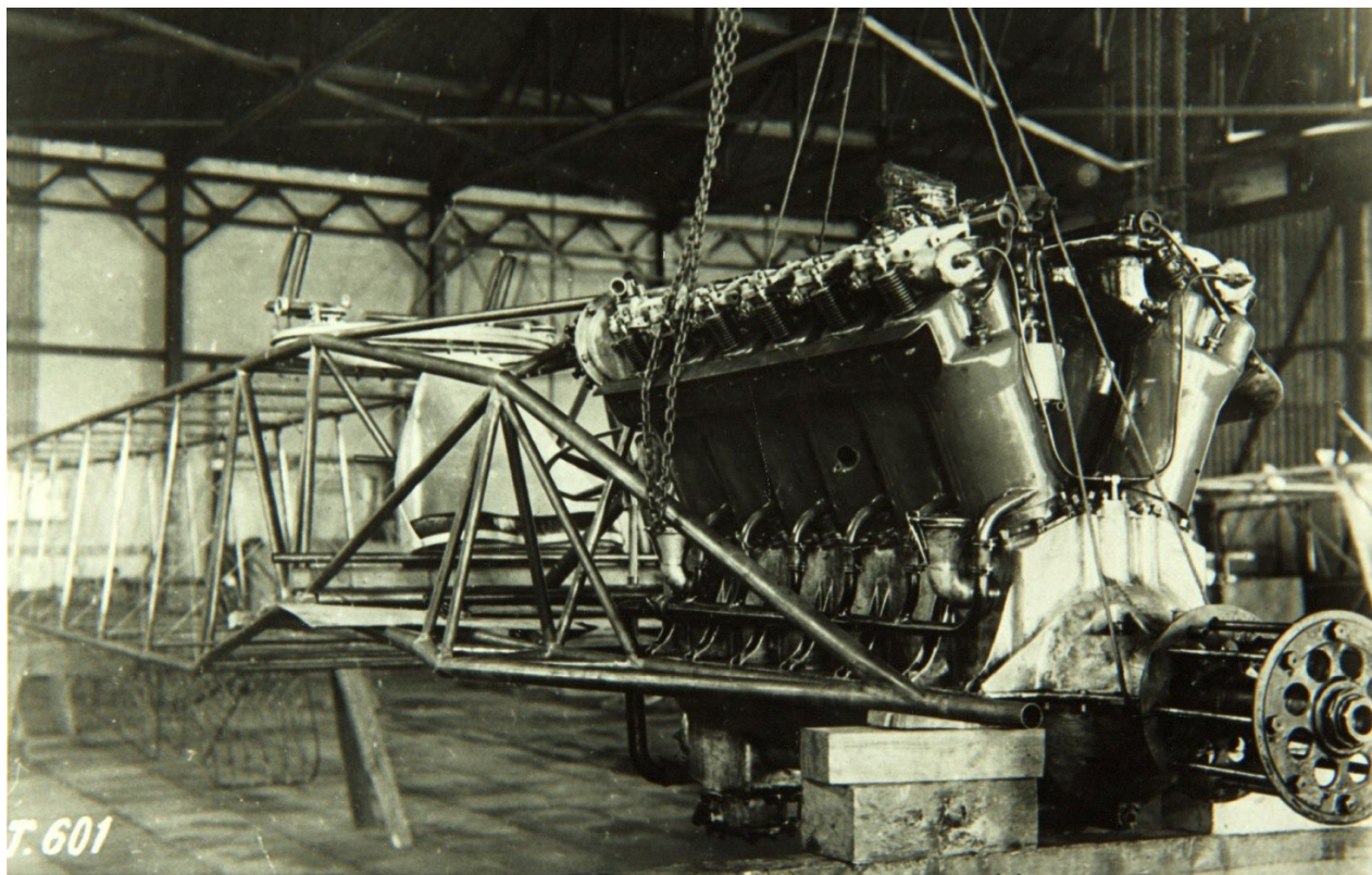
Fokker C.IV en la línea de fabricación
