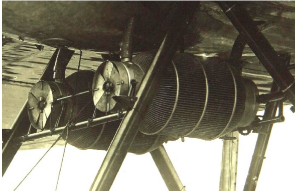
Radiador circular Lamblin
