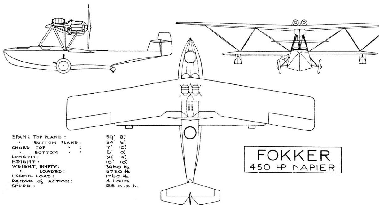
Variante proyectada del Fokker B.II con motor impulsor
